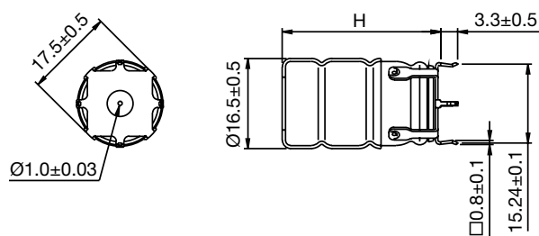
Dimensions table PEH220-226 (mm)
