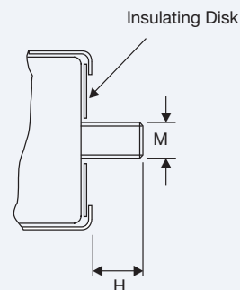
ALS41 Stud Mounting
