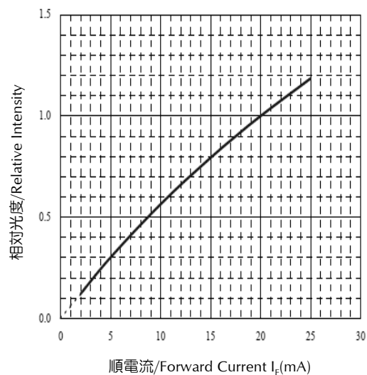
順電流—相対光度 特性
