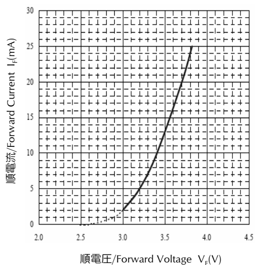
順電圧—順電流 特性
