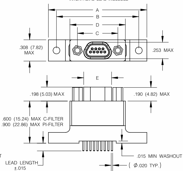
RECEPTACLE
