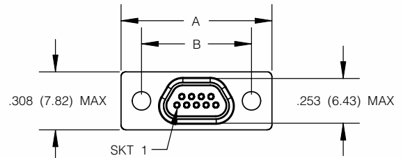
RECEPTACLE
