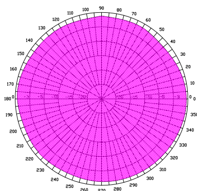
垂直方向图
