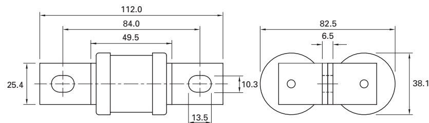
FMM, MMT — indicator optional
