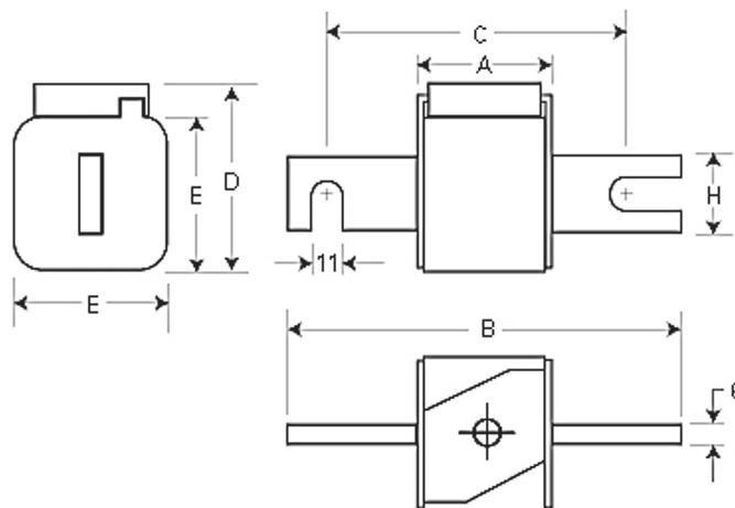
Type -KN/80, -KN/110
