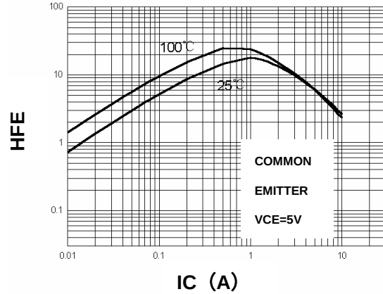
HFE – IC
