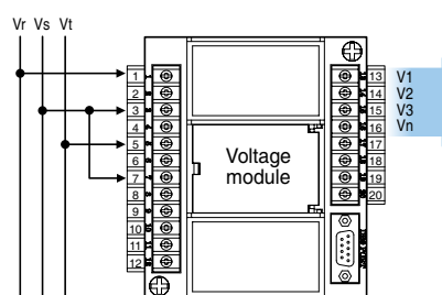
3P3W wiring
