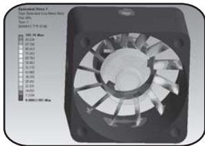
振动模式模拟分析
