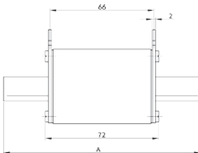
gPV, PV(gR) 750V, 1000V dimensions
